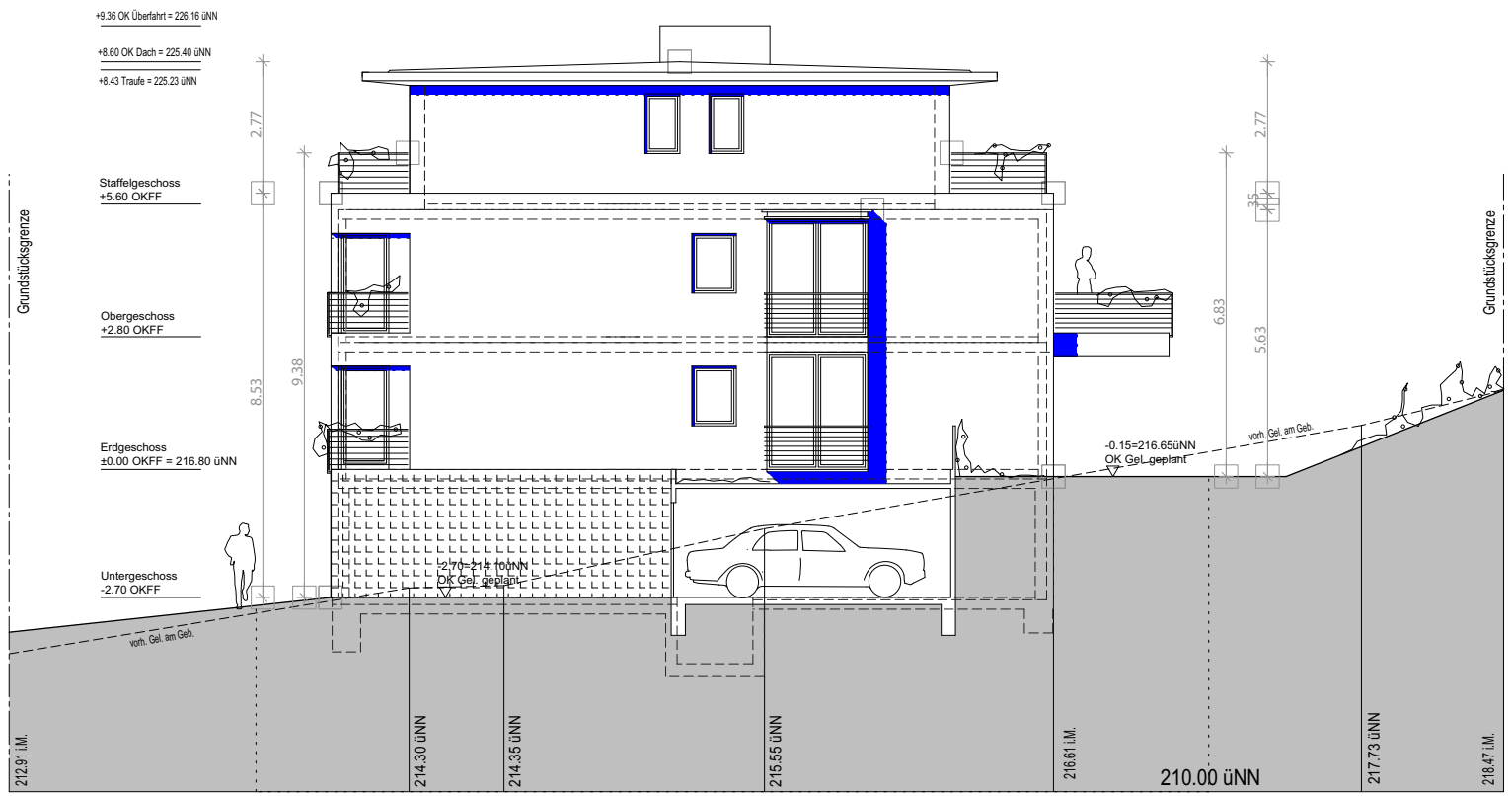
Ansicht Westen
