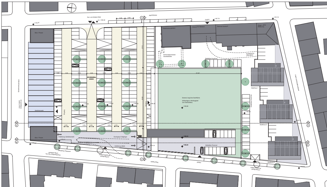
Lageplan M 1: 500
