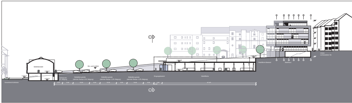
Schnitt A-A M 1: 500
