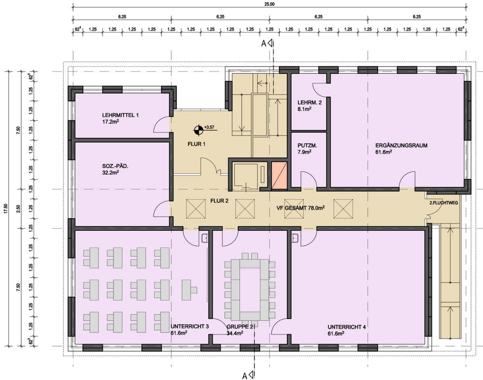
GRUNDRISS OBERGESCHOSS
