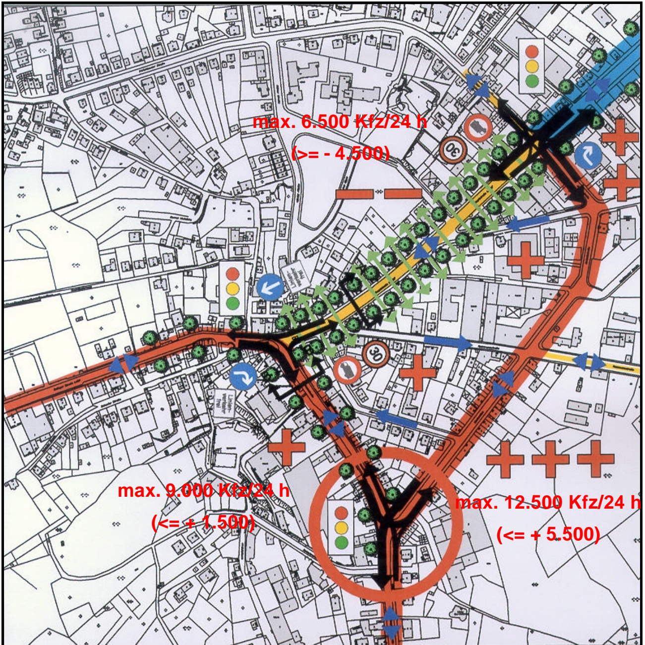
Abb. 6-5: Szenario 4: Verbot der Fahrbeziehungen Solinger Straße – Hauptstraße und Hauptstraße – Rathausstraße
