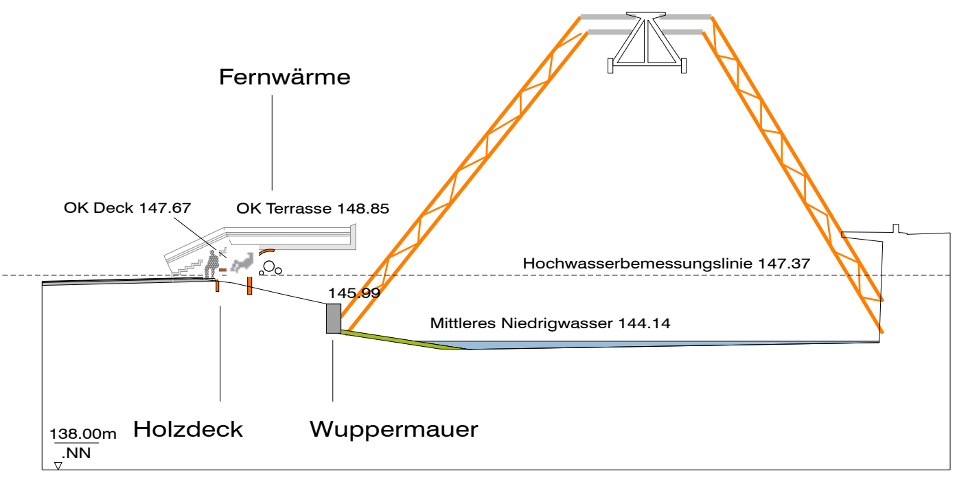
Schnitt C-D
