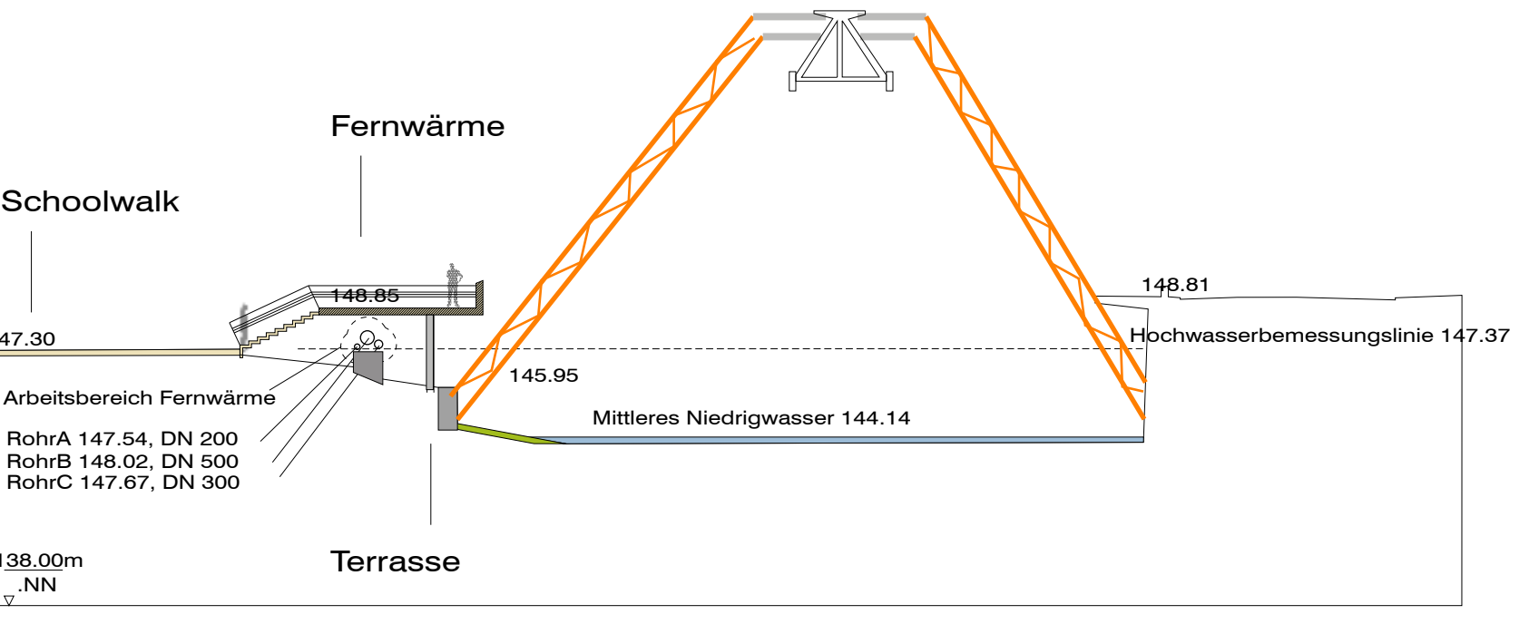
Schnitt A-B
