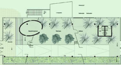
Pflanzenbahnhof Grundriss EG M 1:100
