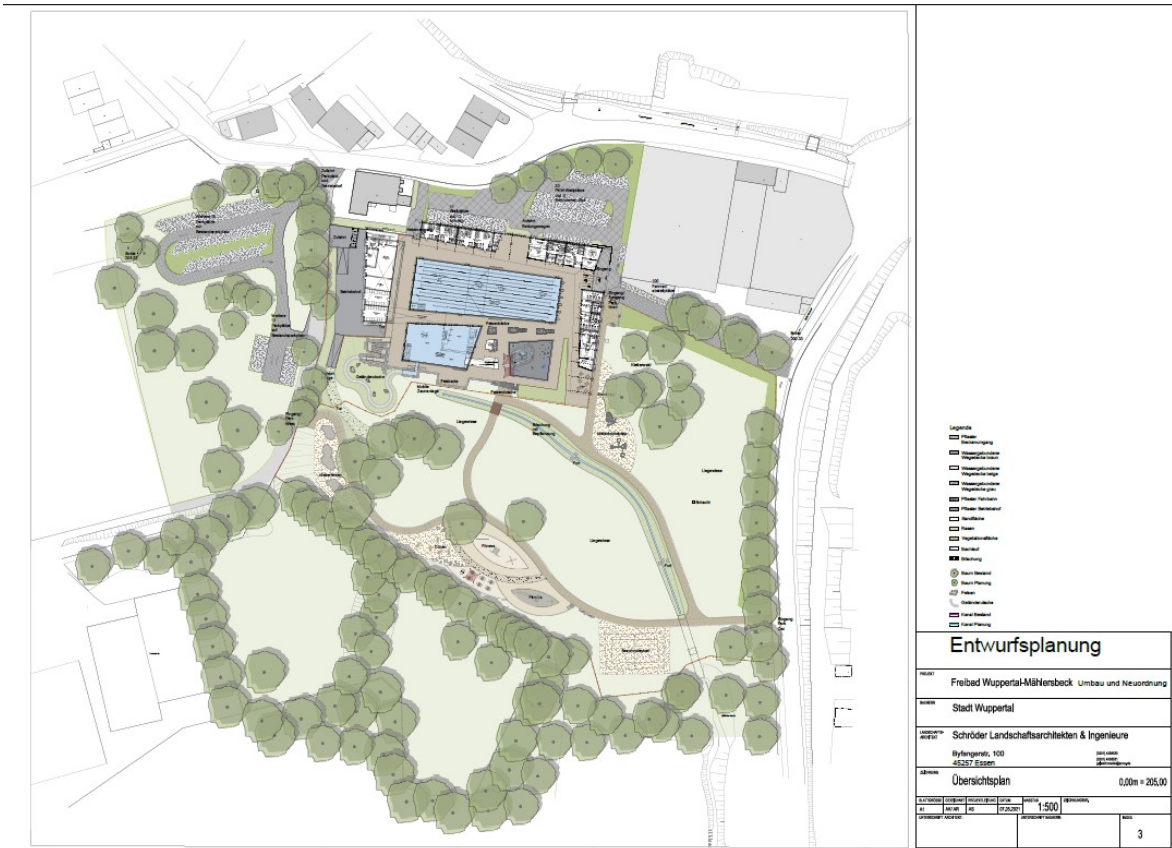
Außenanlagenplan
