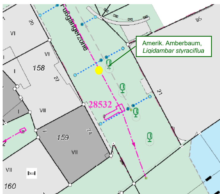
Abb. 1: Lage des geplanten Schachts 53475 (vorh. Schacht-Nr. 28532)
