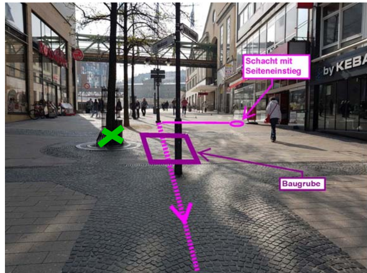
Abb. 3: Lage des Kanals, des vorh. Schachtes und der gepl. Baugrube in der Fußgängerzone
