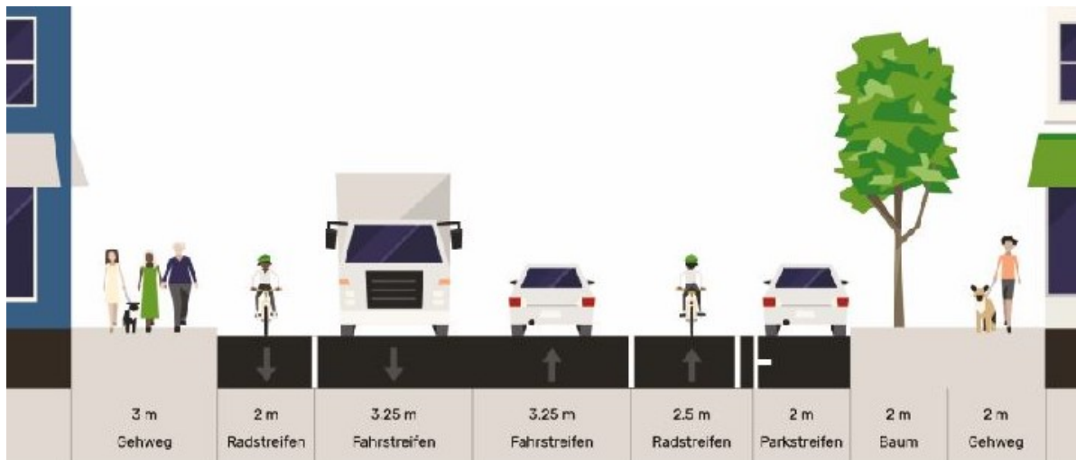
Abbildung 2: Querschnitt Jägerhofstraße Planung, Quelle:Streetmix.net
