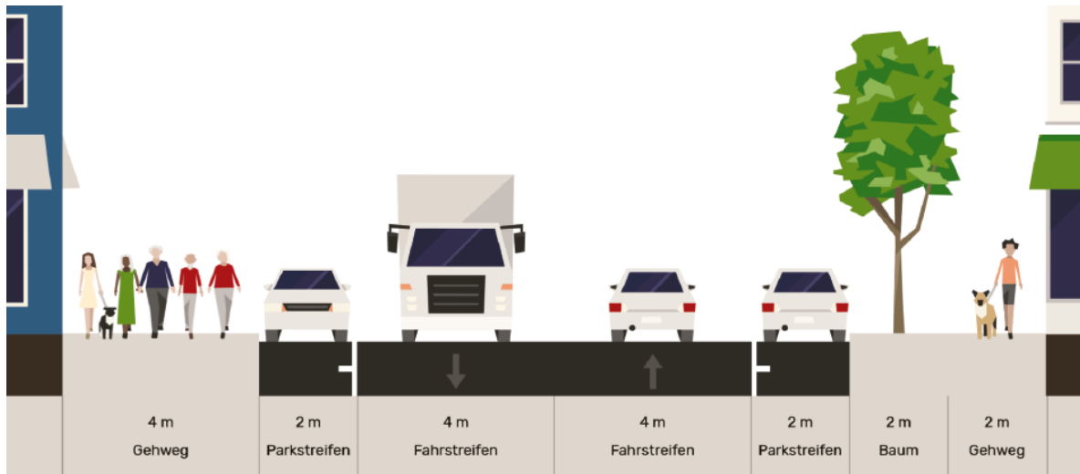
Abbildung 1: Querschnitt Jägerhofstraße Bestand, Quelle:Streetmix.net
