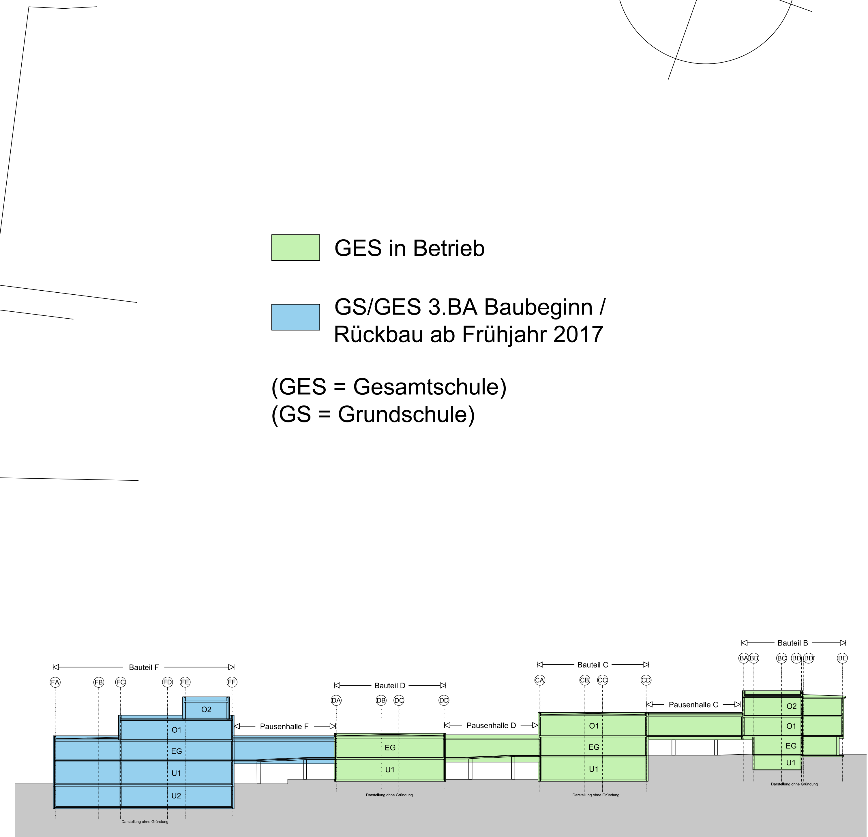
Schnitt
