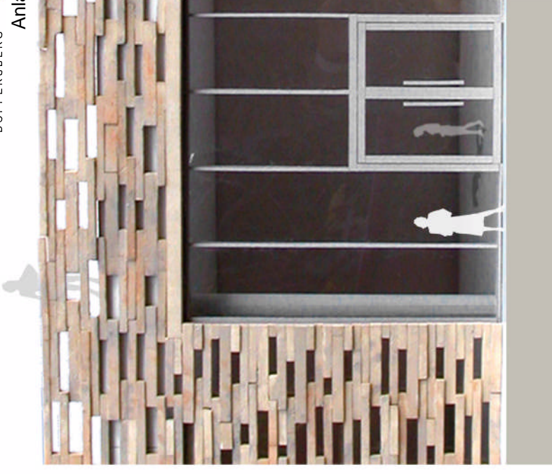
TEILANSICHT NATURSTEIN-/GLASFASSADE M 1:20
