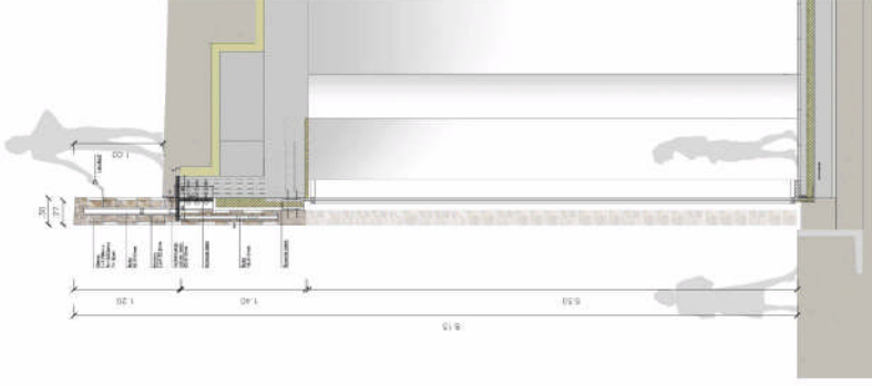
SCHNITT LADEN GLASFASSADE M 1:20
