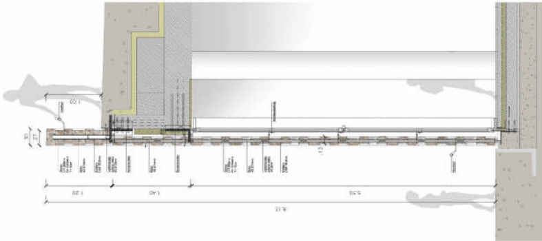
SCHNITT LADEN NATURSTEINFASSADE M 1:20
