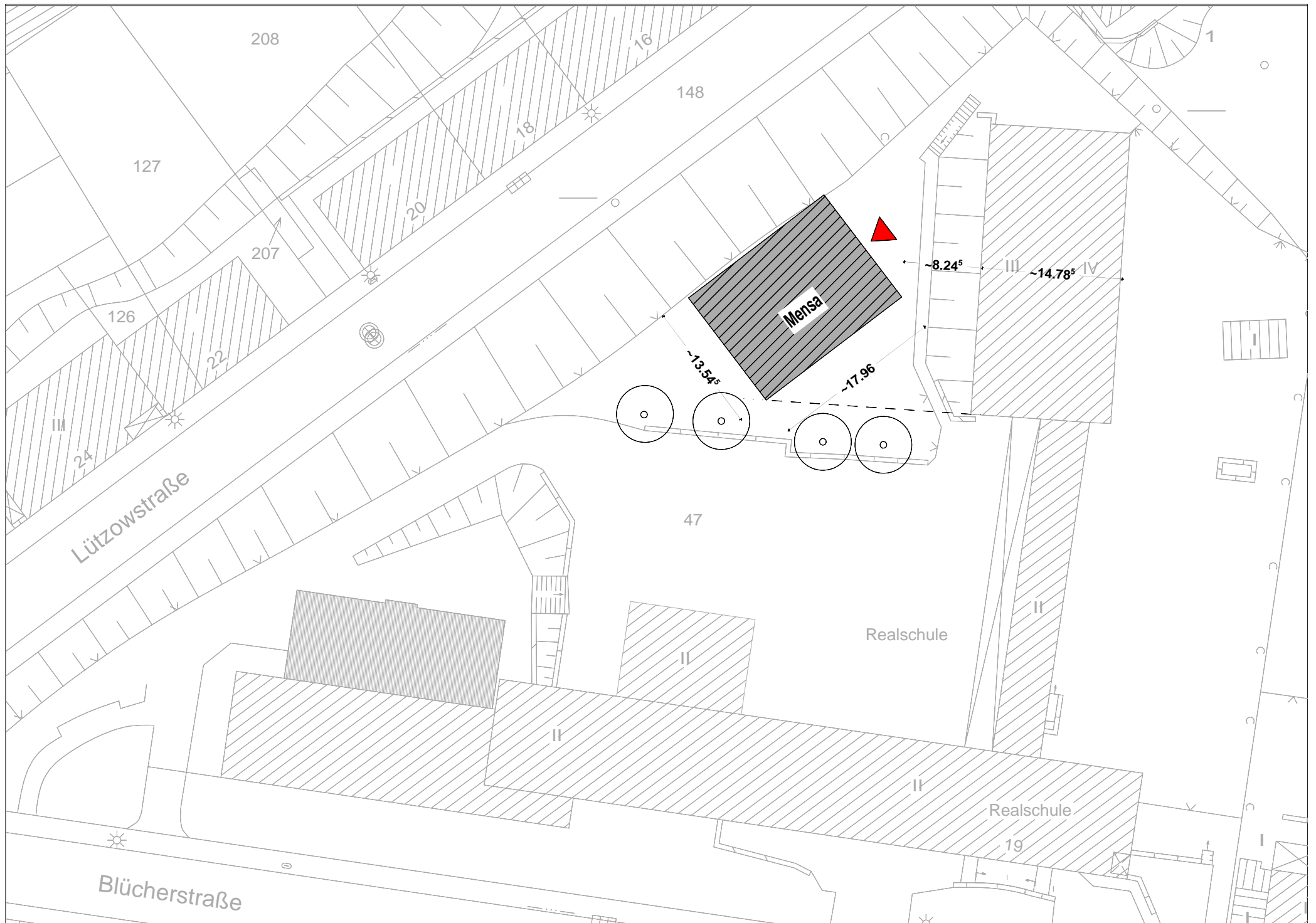
2009-12-17 Lageplan Blücher - M 1:500
