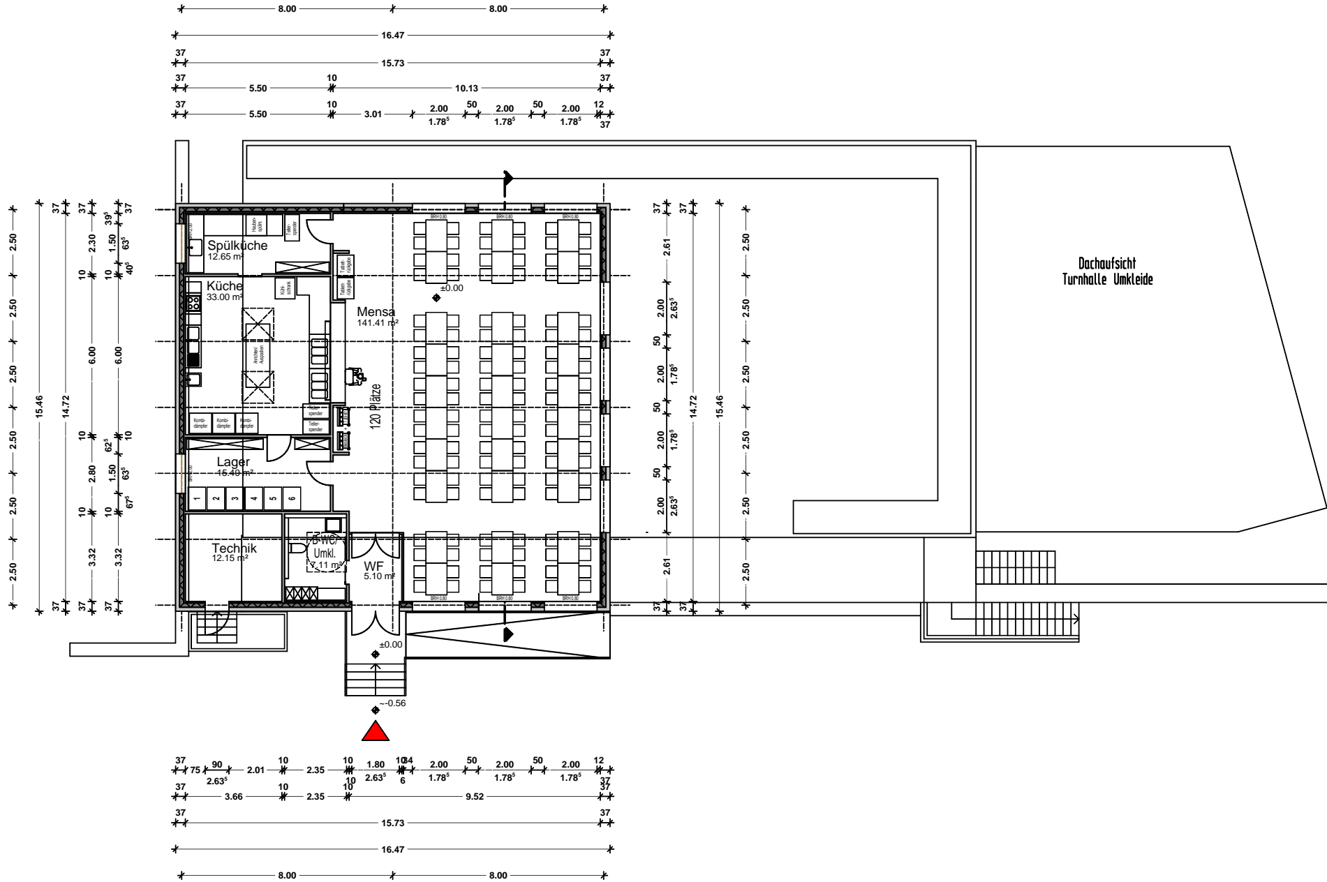
Grundriss Mensa Sedanstraße - M 1:200
