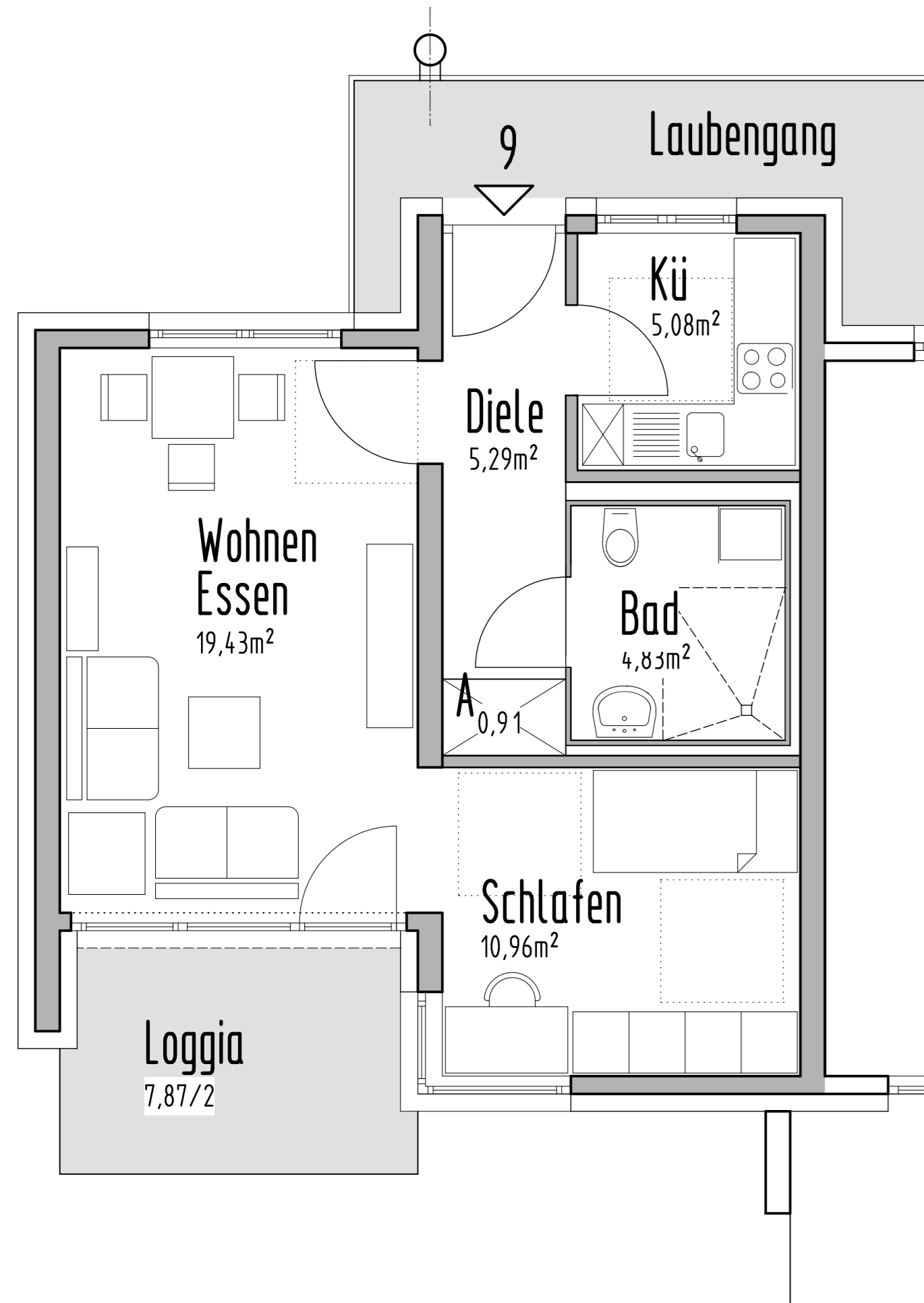
WHG Typ A Wohnfl. 50,44 m 2
