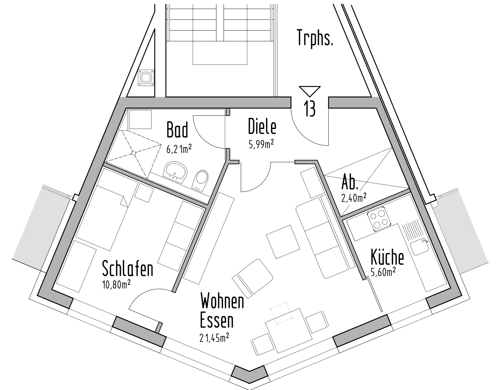
WHG Typ C Wohnfl. 52,45 m 2
