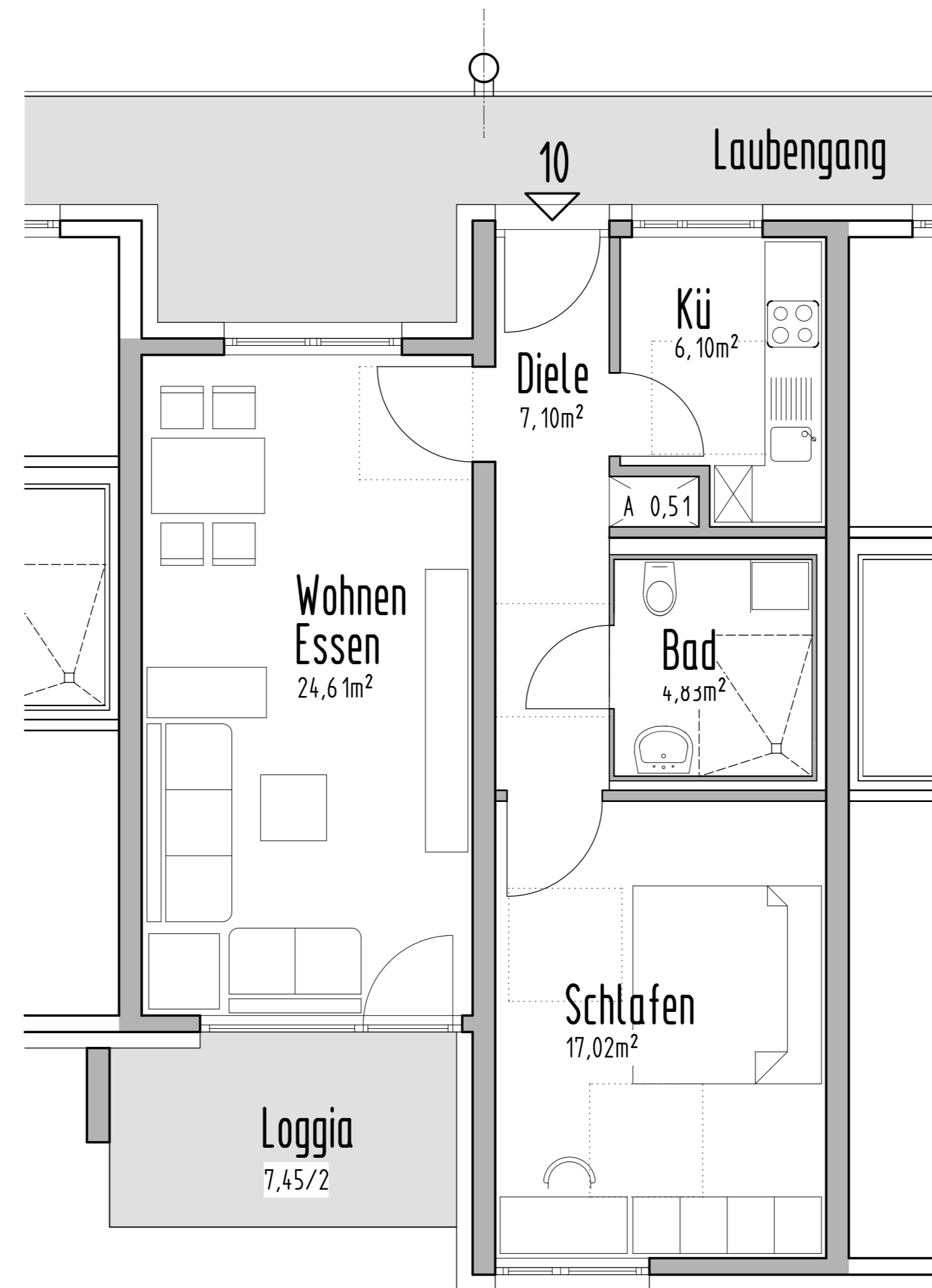
WHG Typ B Wohnfl. 63,90 m 2
