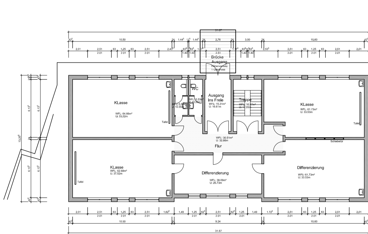
OBERGESCHOSS
