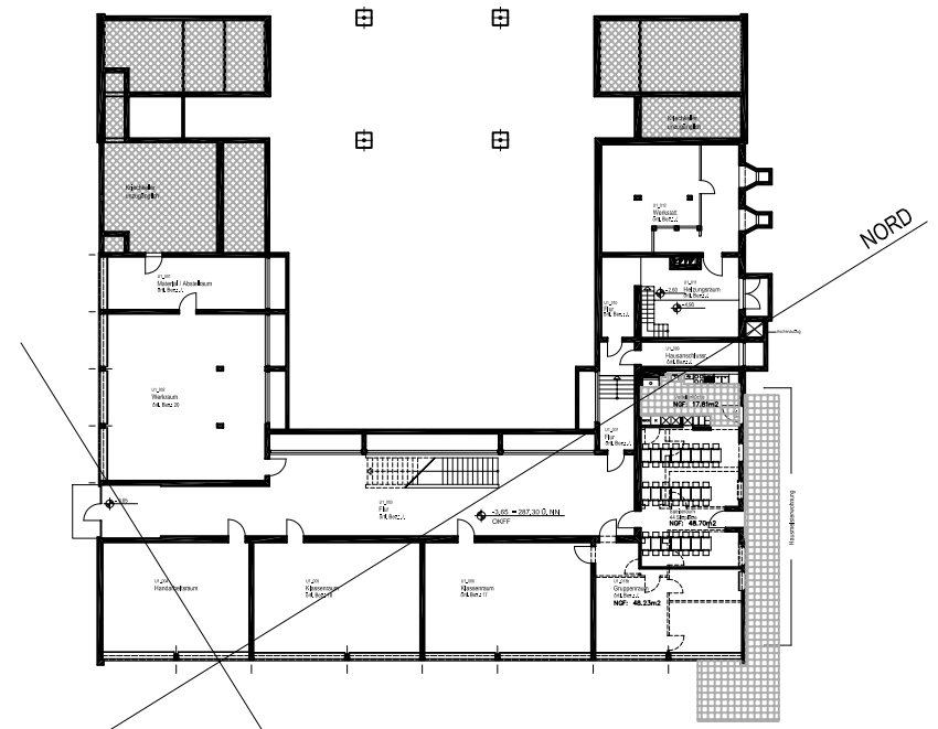
Grundriß UG - M 1:500 Verteilerküche + Speiseraum / HM-Wohnung
