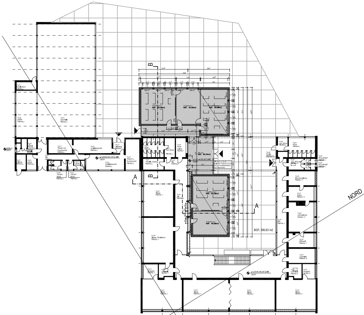
Grundriß EG - M 1:500
