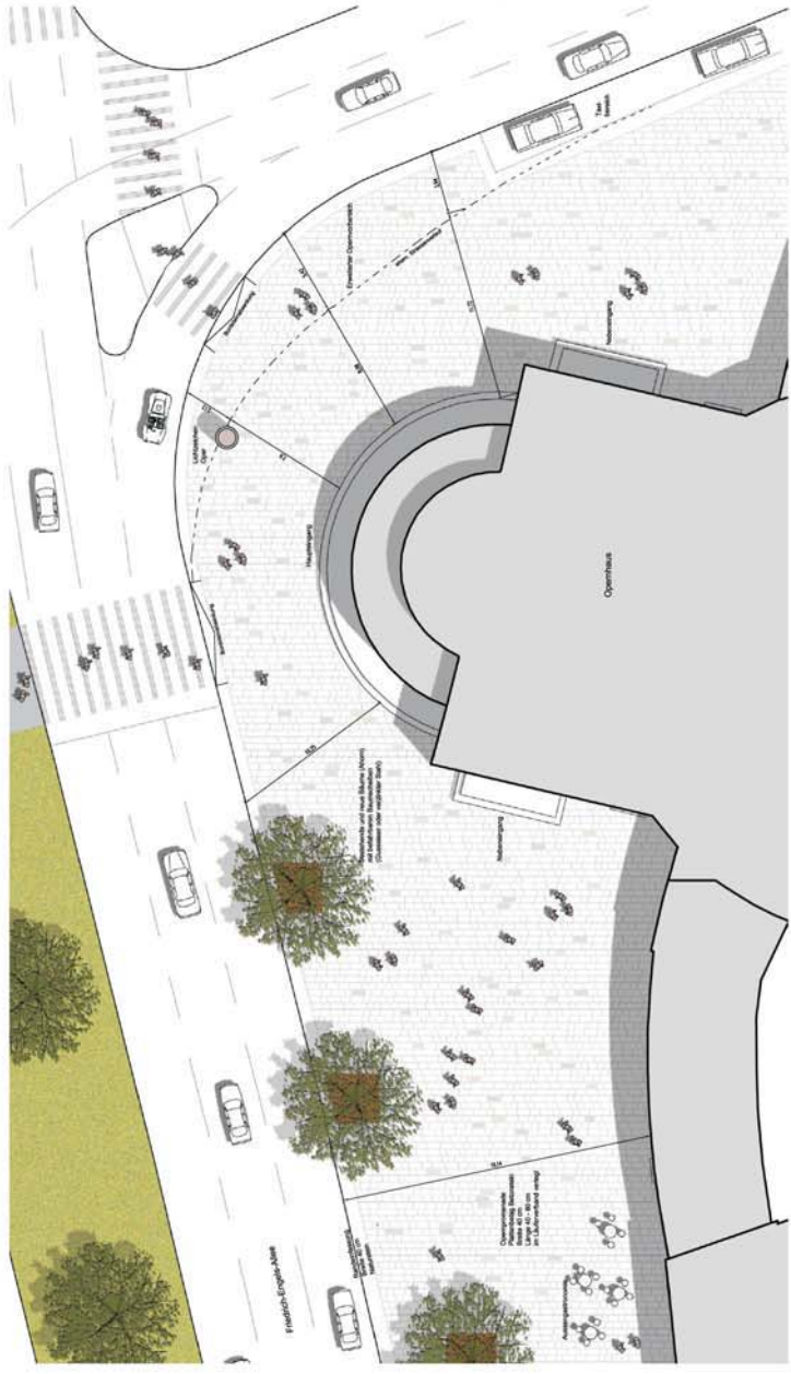
Grundriss Operrampende 1:100
