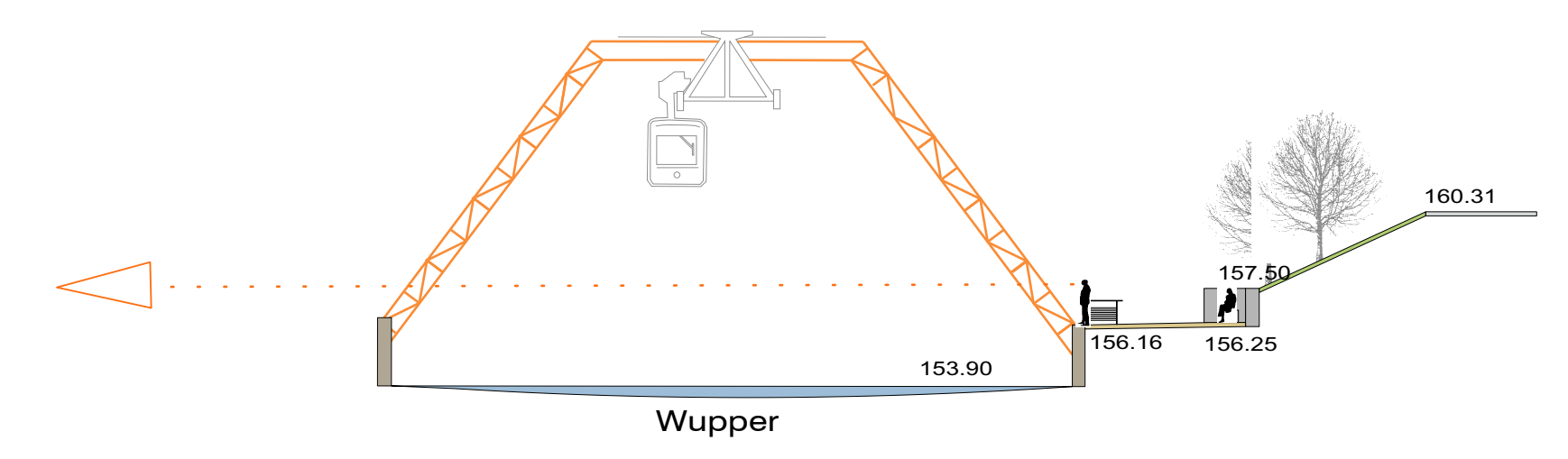
Schnitt C-D
