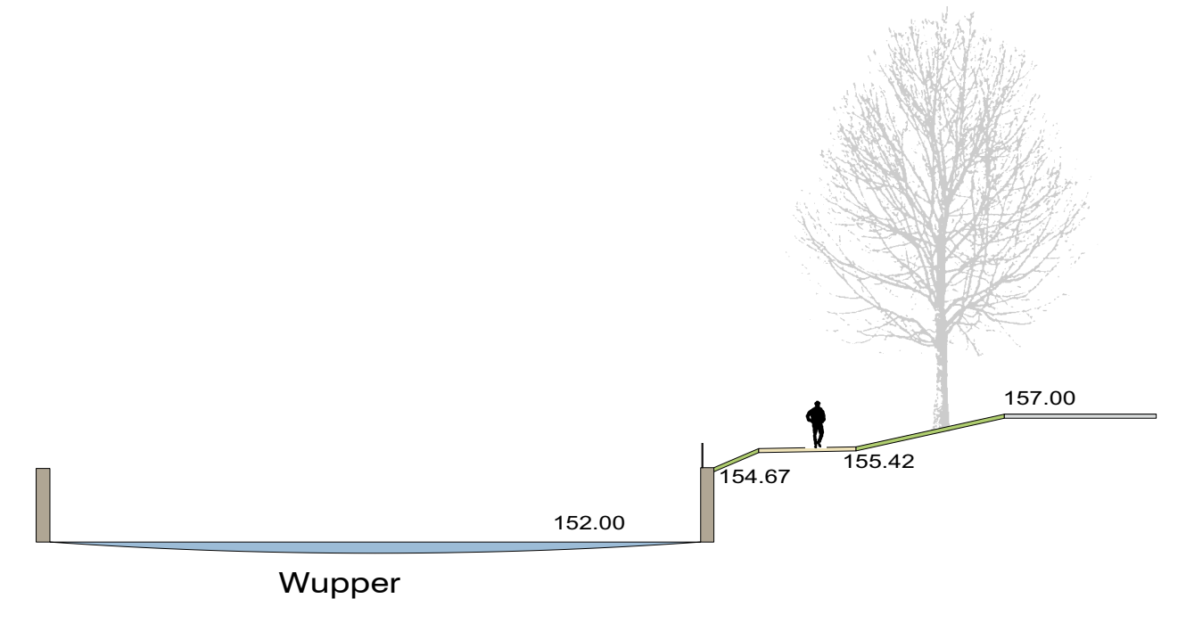
Schnitt A-B
