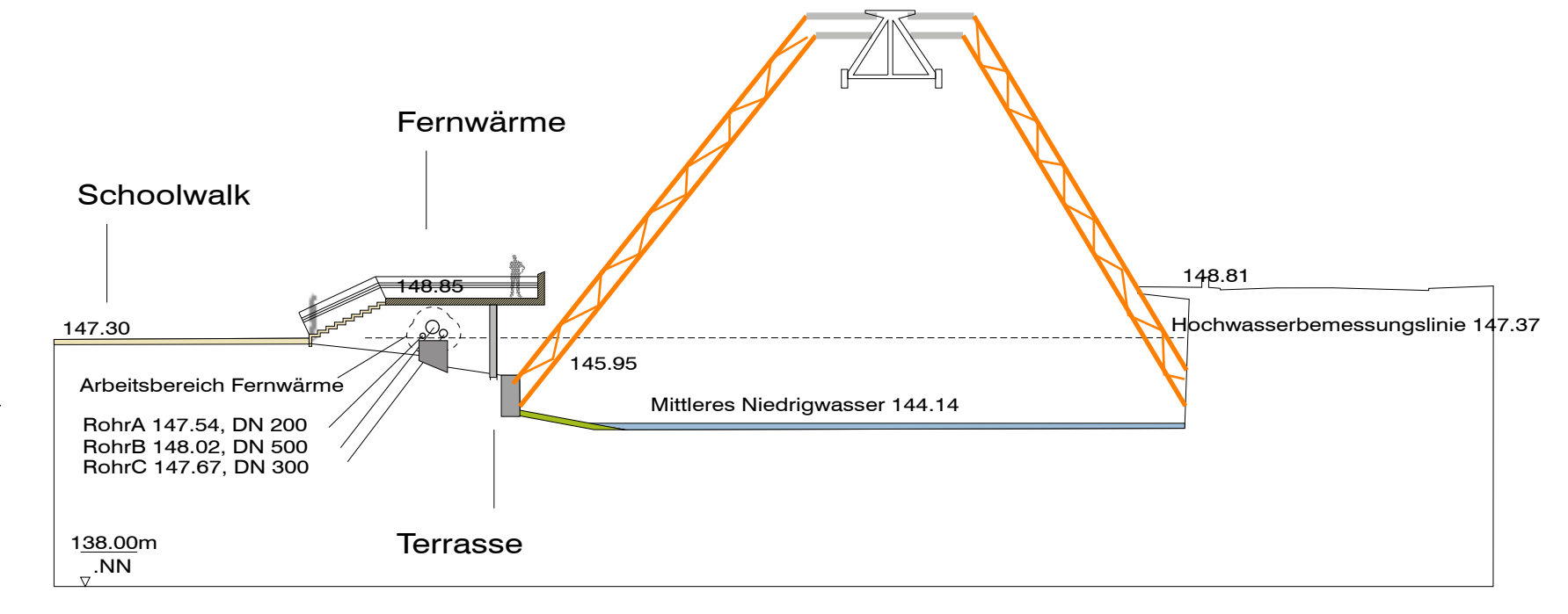
Schnitt A-B
