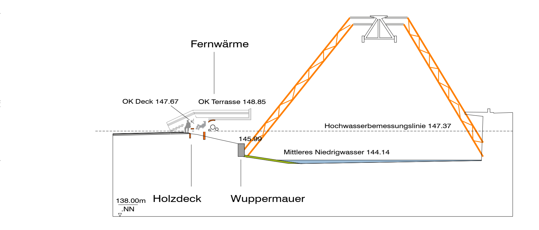
Schnitt C-D
