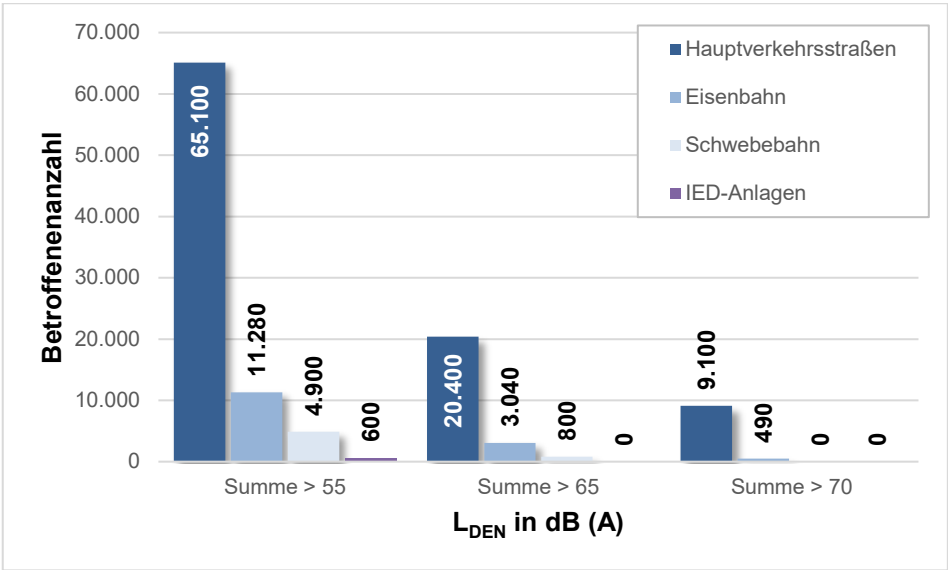
Abbildung 6: Betroffenenvergleich zwischen den Lärmverursachern im Tagesmittel (L DEN )
