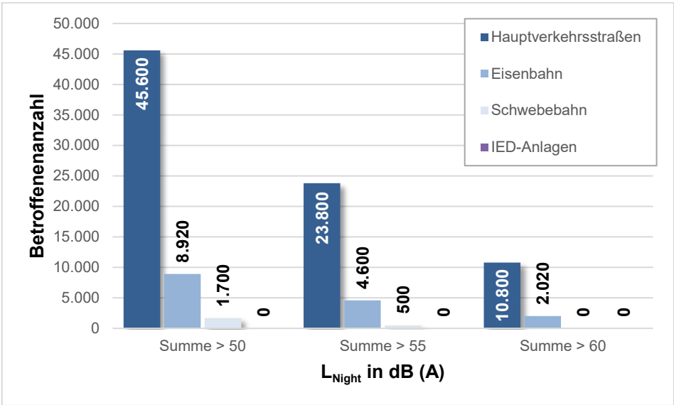
Abbildung 7: Betroffenenvergleich zwischen den Lärmverursachern in den Nachtstunden (L Night )
