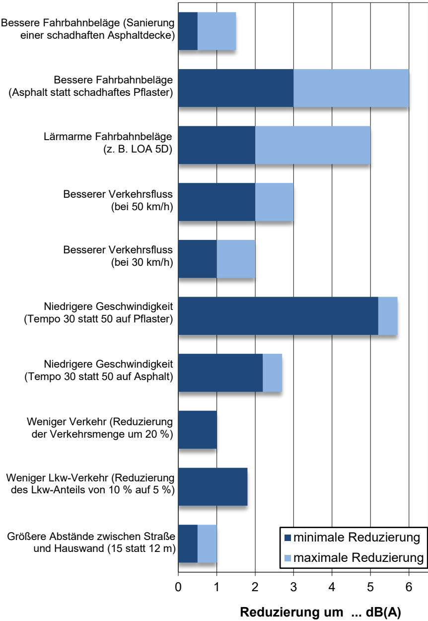
Abbildung 12: Lärminderungspotenziale ausgewählter Maßnahmen
