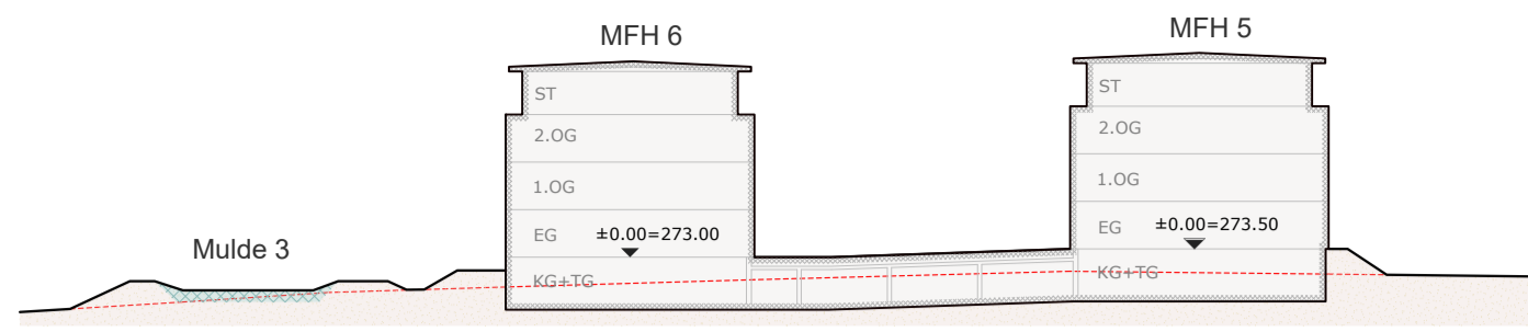
Schnitt D/D
