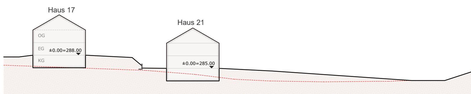
Schnitt E/E
