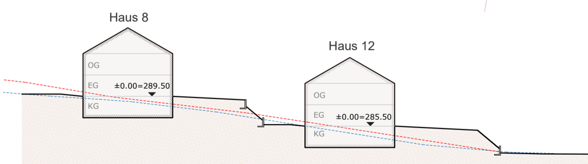
Schnitt F/F
