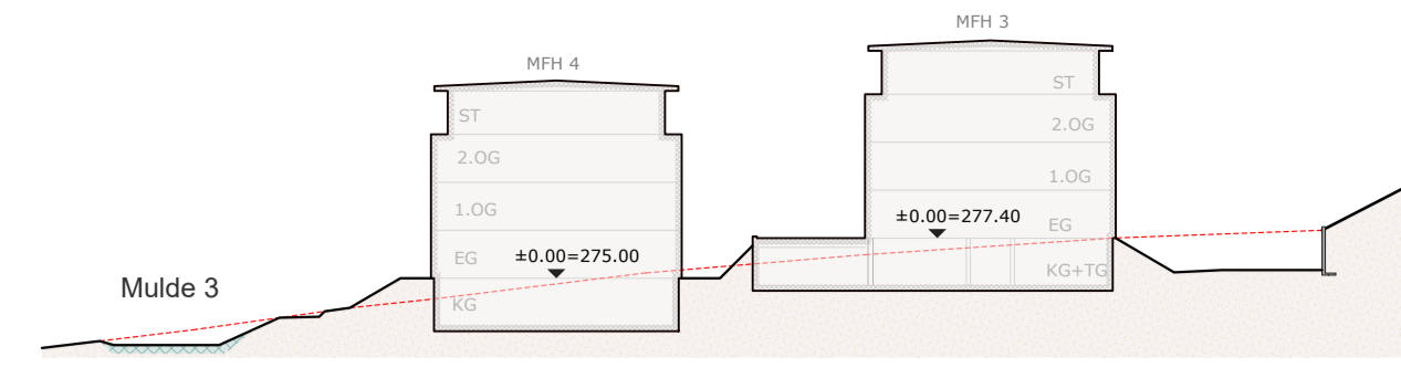
Schnitt B/B
