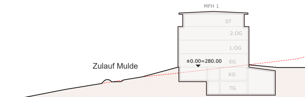
Schnitt A/A
