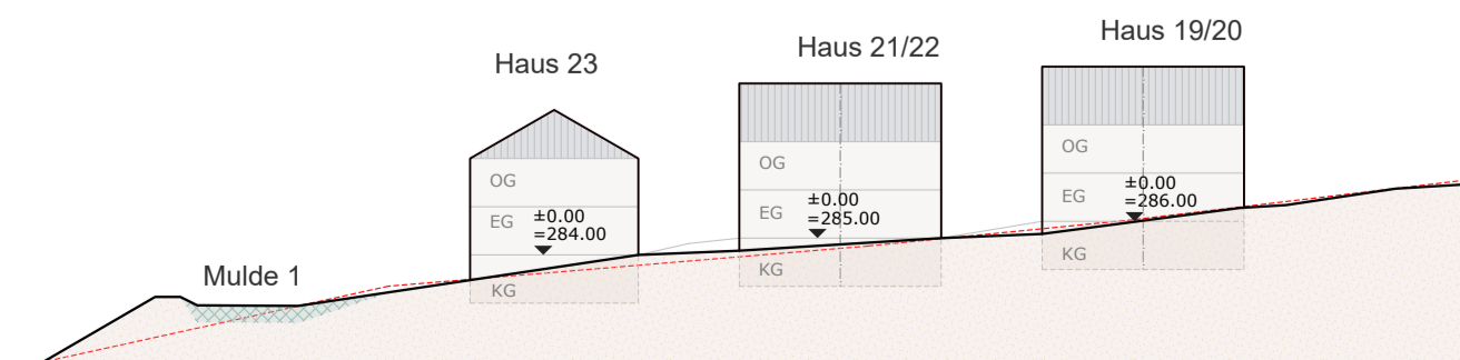
Schnitt H/H
