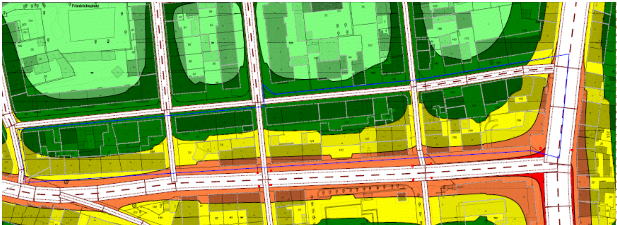
Abb. 8: Lärmberechnung gem. DIN 4109 nachts (22 – 6 h)
