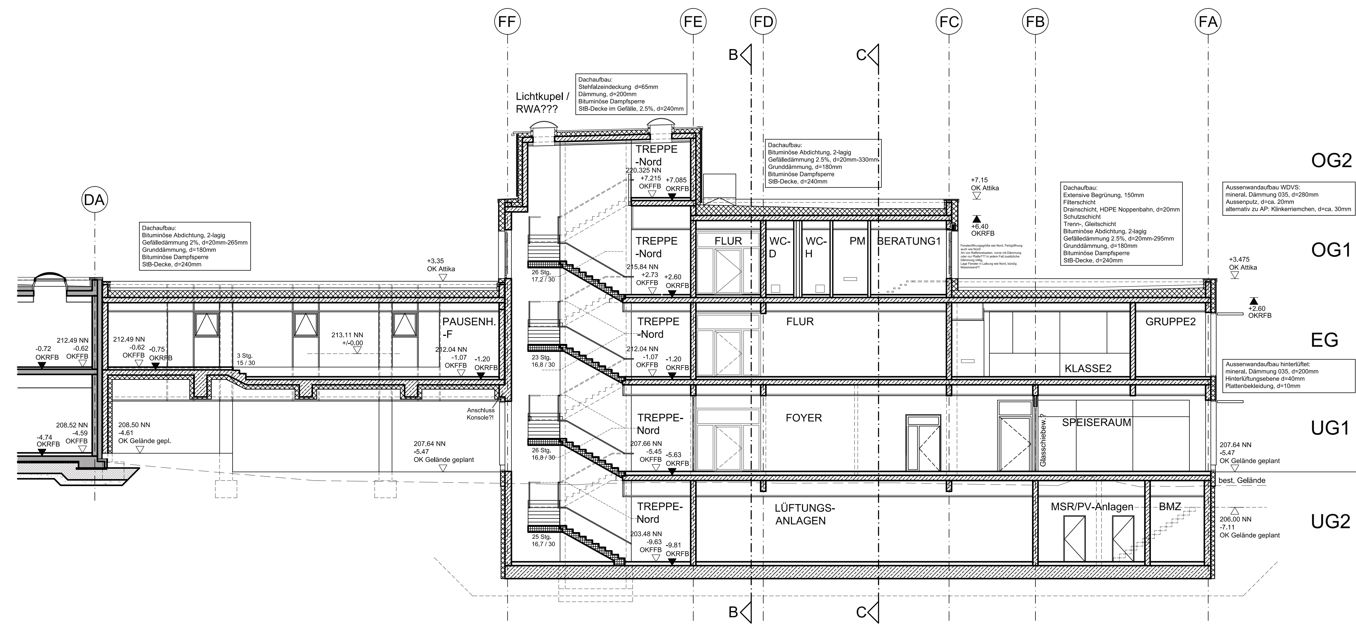
SCHNITT A-A
