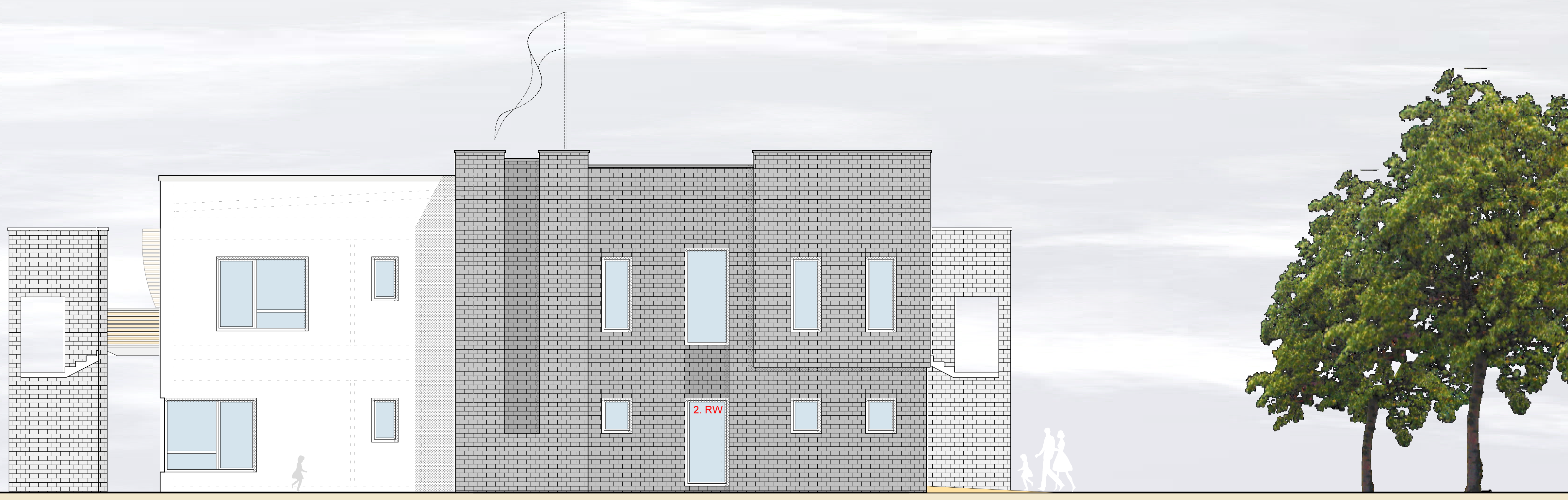
ANSICHT SÜD
